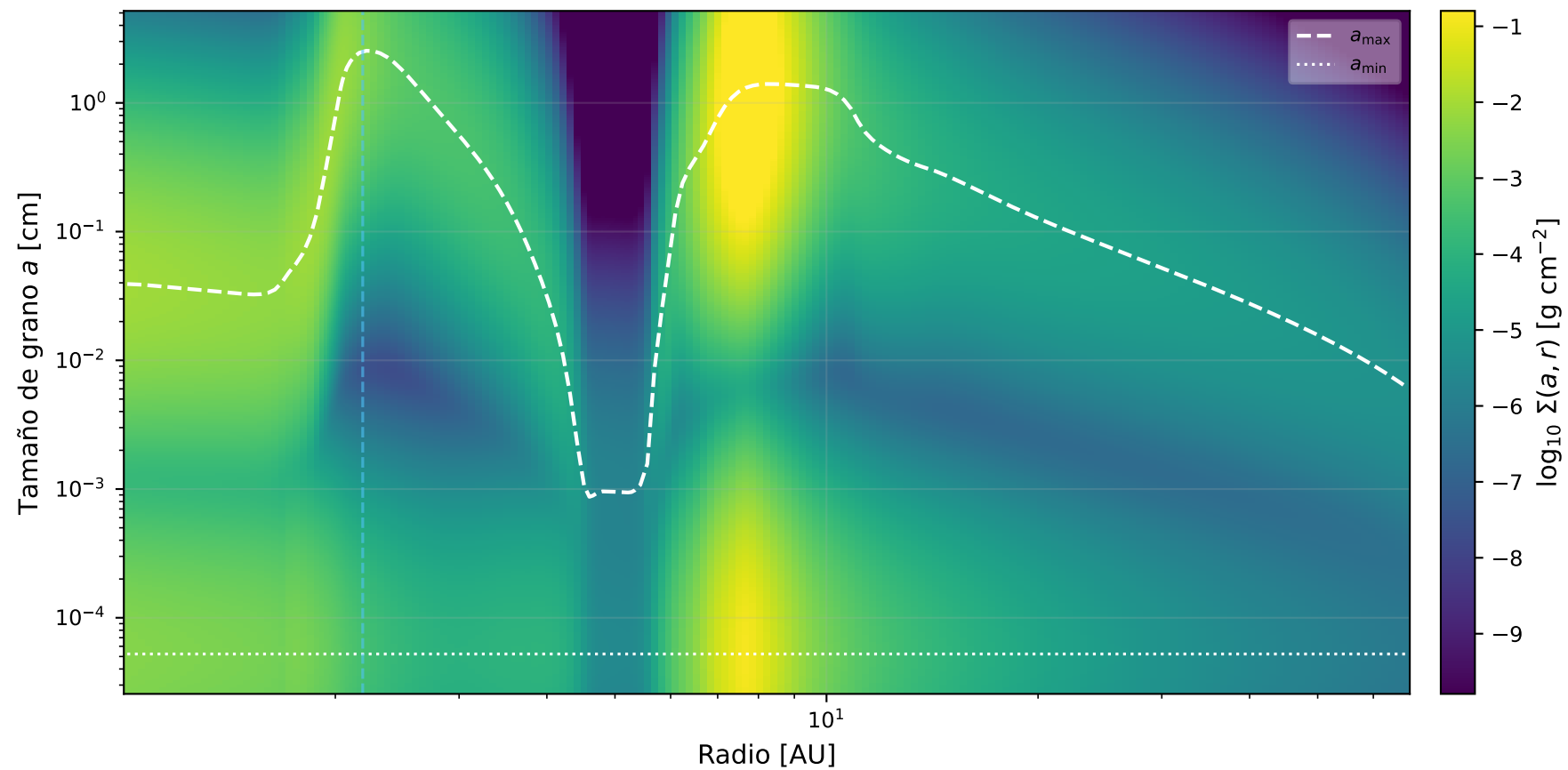
Distribución de tamaño de grano vs radio | t = 2.88\text{e}+06 yr
